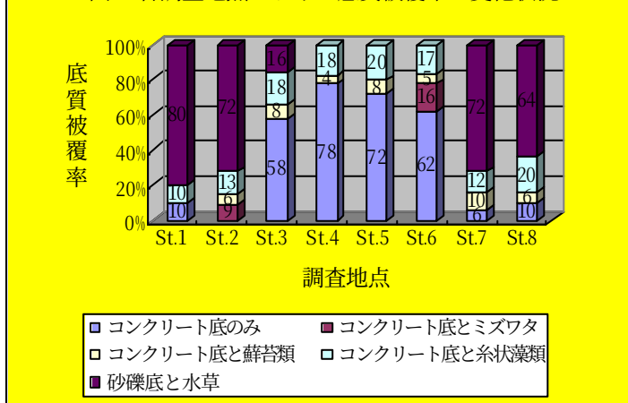
図4 各調査地点における底質被覆率の変化状況
