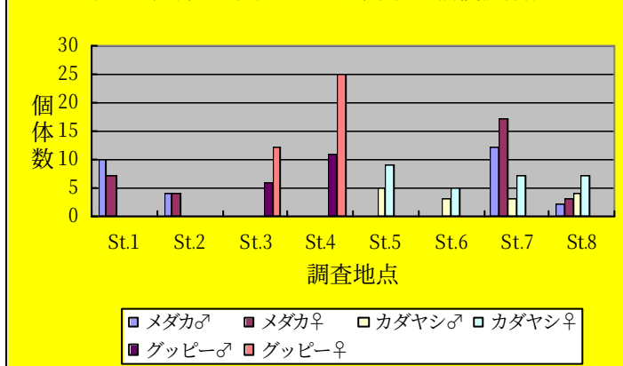
図3 各調査地点における対象種の捕獲個体数
