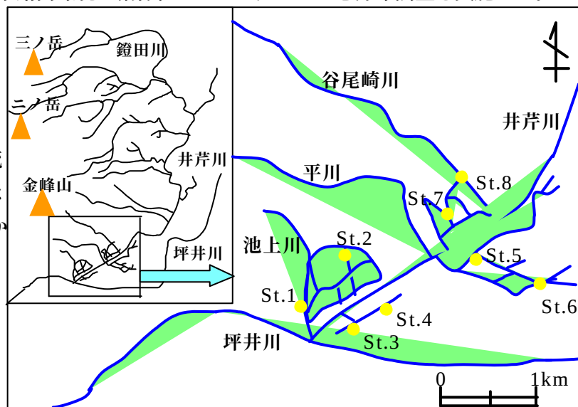
図1 調査地点概略図
