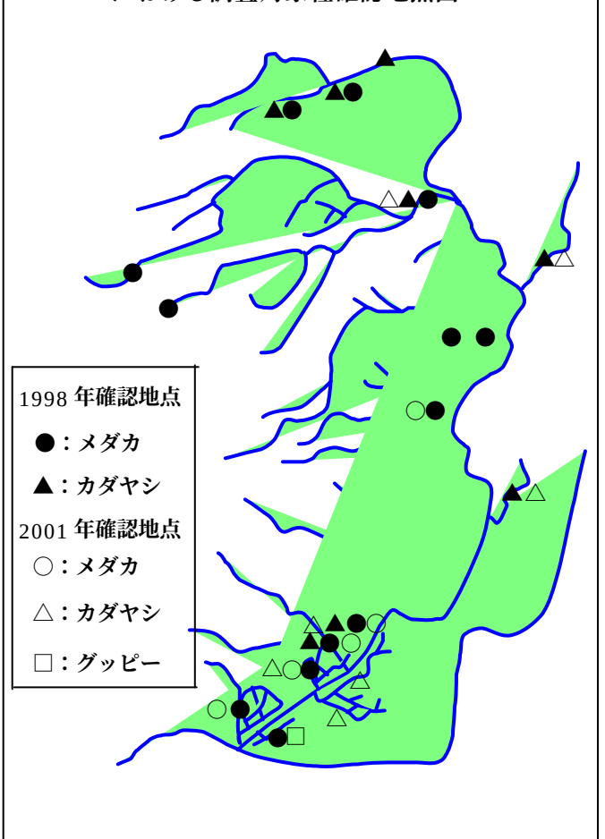
図2 現地調査(1998年及び2001年)における調査対象種確認地点図
