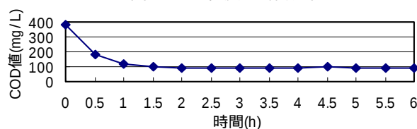
図-5 COD値の時間変化
