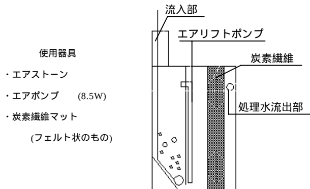
図-3 活性汚泥処理装置
