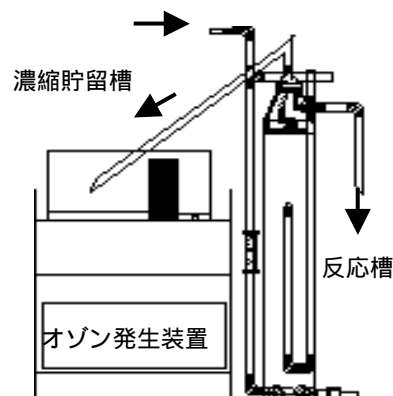
図 - 3 装置図
