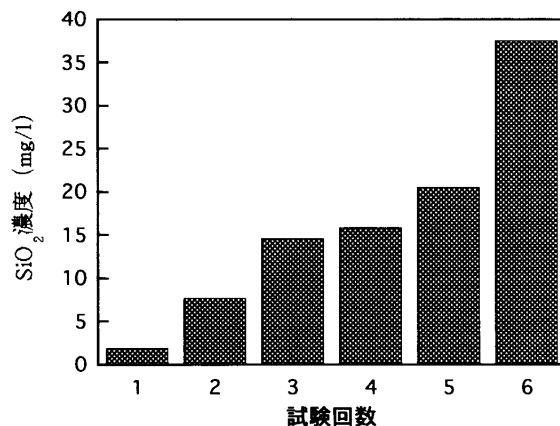
図4 スラグの繰り返し溶出試験における試験回数に伴う検水中のケイ酸濃度の変化
