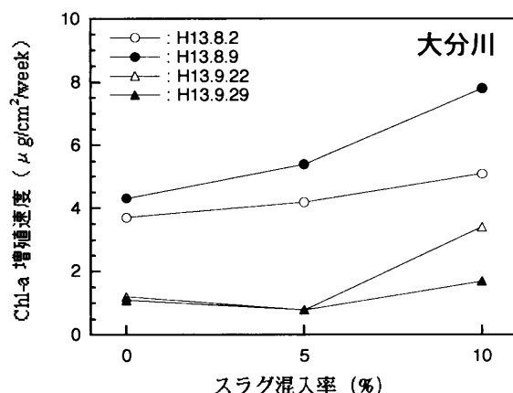
図2 大分川に設置したスラグブロック（半球形）におけるスラグ混入率と付着藻類増殖速度の関係
