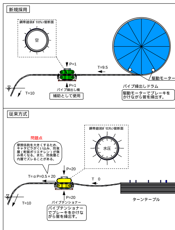
図 - 3 繰出し方法比較図
