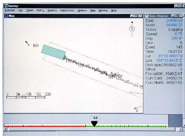
図 - 4 敷設船位置管理状況
