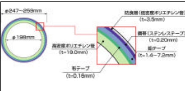
図－2 鋼帯鎧装ポリエチレン管構造図
