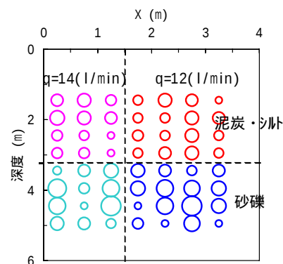
図4 貫入試験結果(従来工法)
