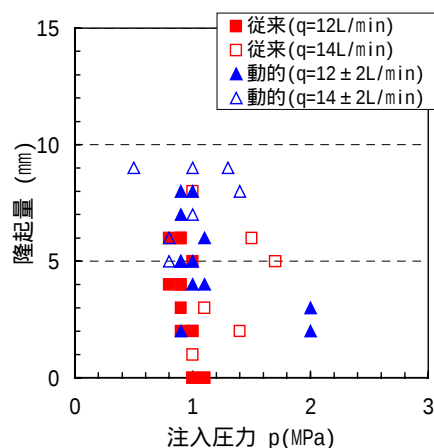
図6 地盤隆起と注入圧力
