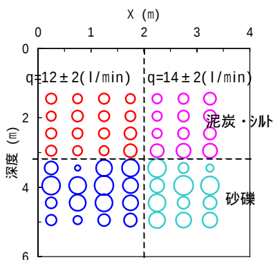
図3 貫入試験結果(動的注入)
