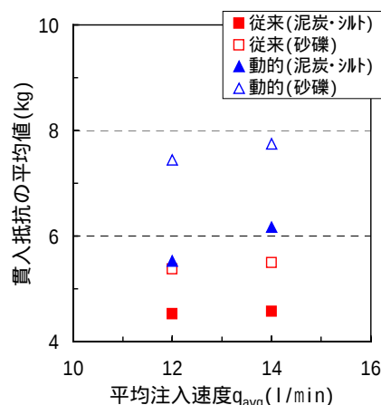
図5 貫入試験結果の平均値
