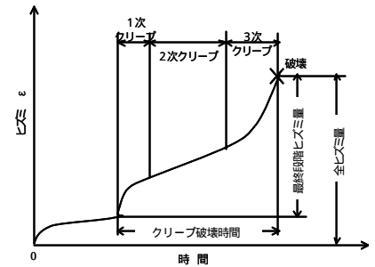
図-3 クリープ曲線
