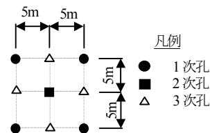
図-1 孔配置図
