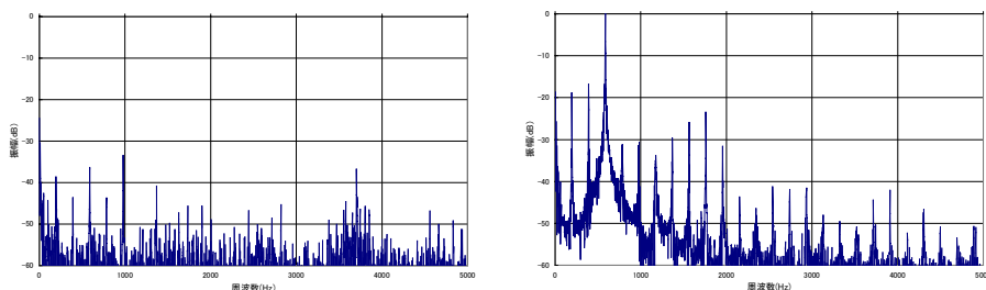
図 1 受信波の FFT 解析例（左：健全部、右：劣化・空洞部）
