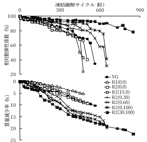
図-1 再生粗骨材の処理方法が凍結融解抵抗性に及ぼす影響
