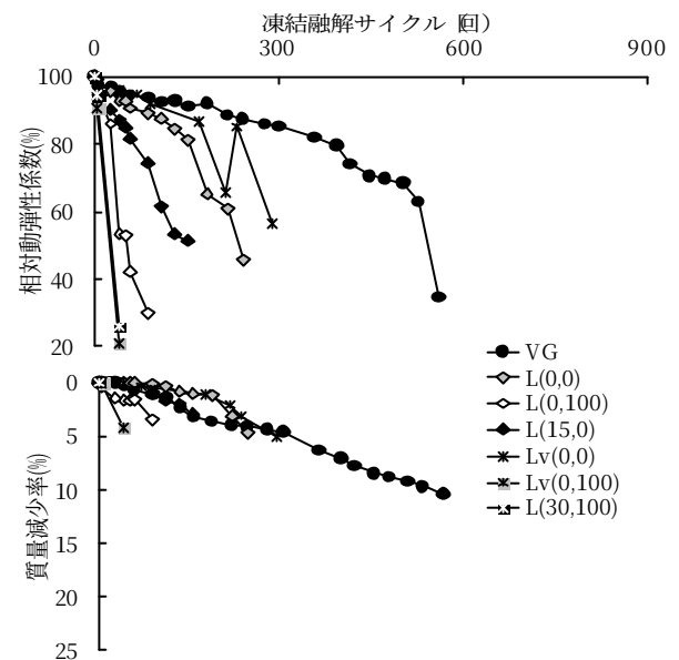
図-2 人工軽量粗骨材の処理方法が凍結融解抵抗性に及ぼす影響
