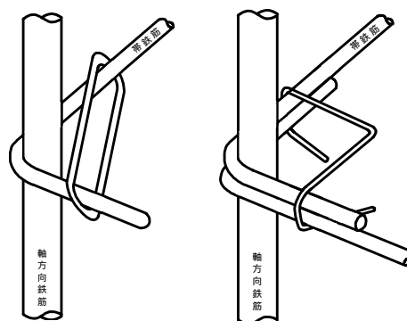
図-2 軸方向鉄筋への定着
