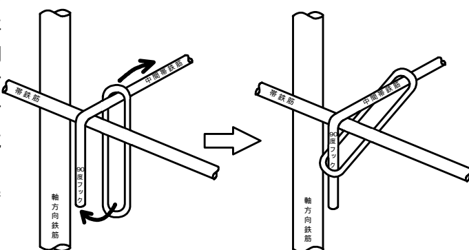
図-1 長円形状のリングによる定着
