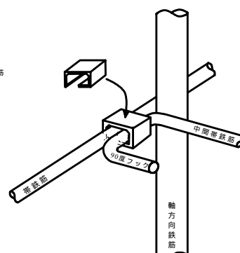
図 - 5 定着金具による 帯鉄筋への定着
