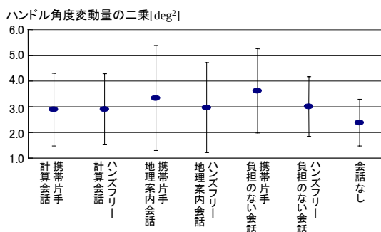
図7.ハンドル角度変動量の二乗の平均
