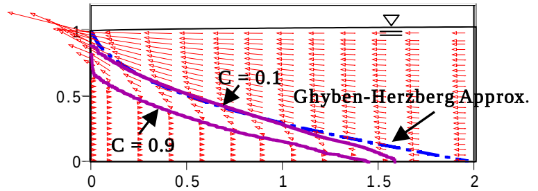
図 - 2 FEM シミュレーションと Ghyben-Herzberg 近似の比較
