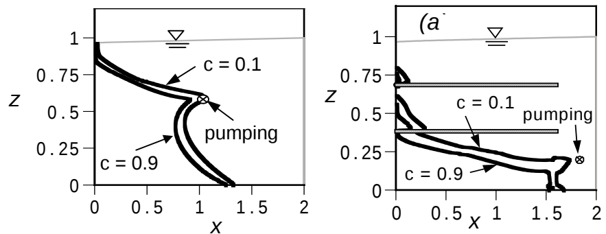
図 - 3 取水時の塩水侵入
