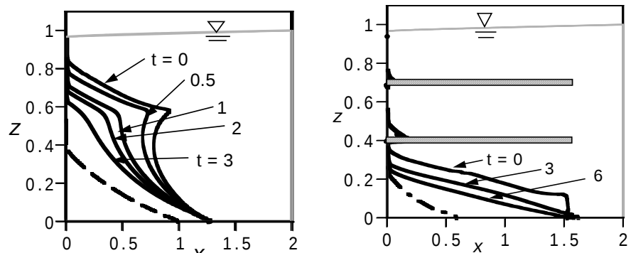
図 - 4 塩水くさびの退行
