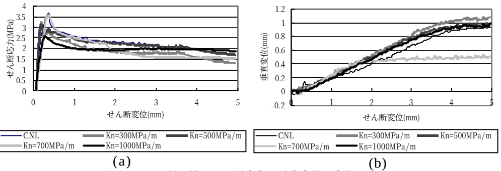
図-3 せん断に伴うせん断応力と垂直変位の変化 ( \sigma_n=1\text{MPa} )
