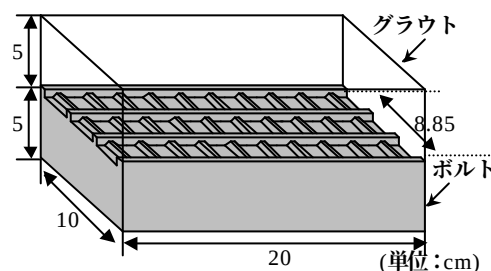
図-2 一面せん断に用いる供試体
