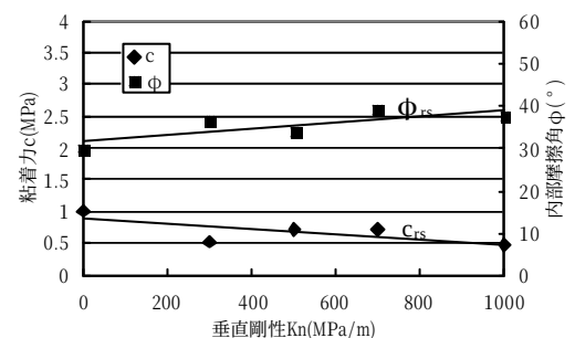
図-6 残留強度における C_r , \phi_r の比較
