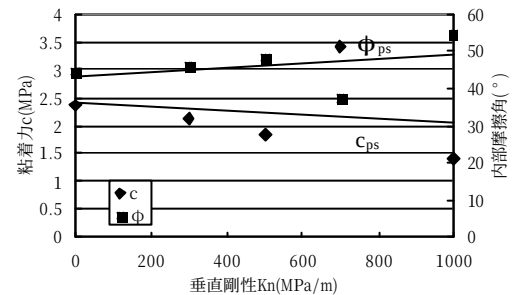
図-5 ピーク応力時の C_p , \phi_p の比較
