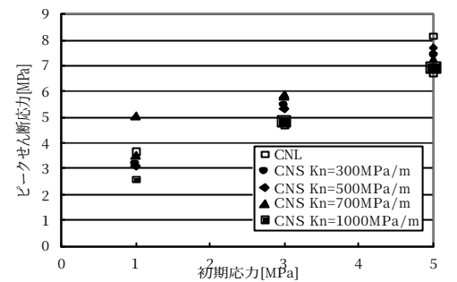
図-4 ピークせん断応力の比較
