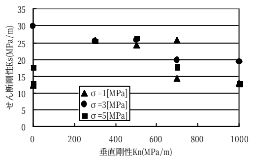
図-7 せん断剛性の比較
