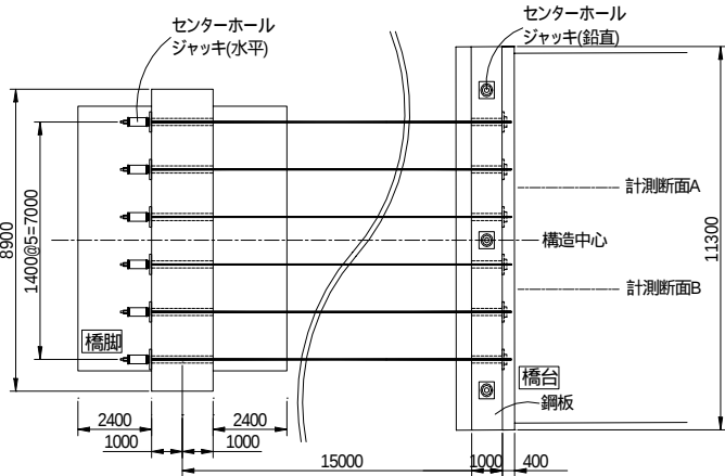
図1 水平載荷試験装置（平面図）
