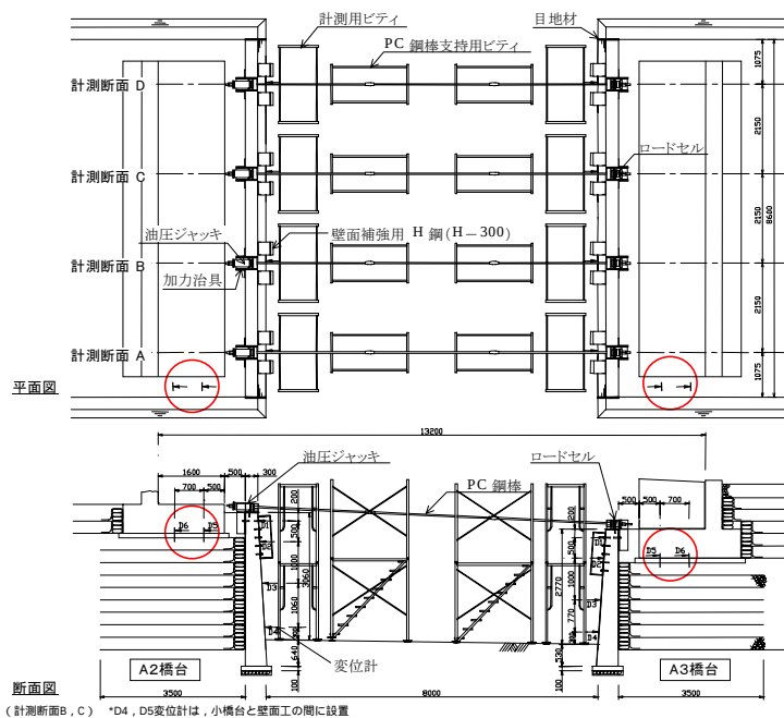
図2 水平載荷試験機器の配置図
