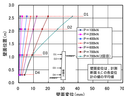
図6 変形モード（A3橋台）
