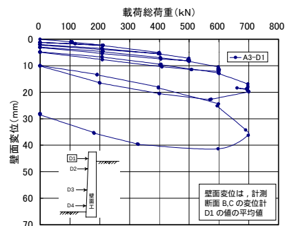
(a) 壁頂部
