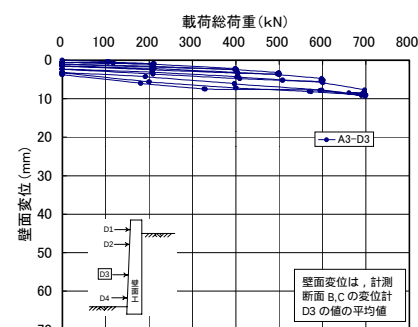
(b) 中間部
