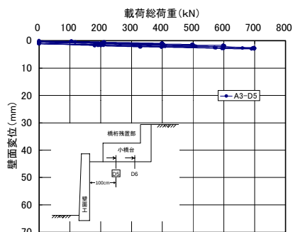
図7 背面盛土の変位（A3橋台）
