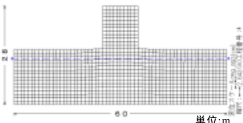
図-6 直下改良地盤変形図
