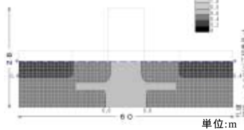
図-3 未改良地盤 F_L 値コンター図
