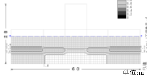
図-5 全面改良地盤 F_L 値コンター図
