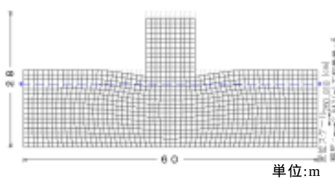
図-2 未改良地盤変形図
