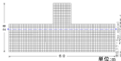
図-4 全面改良地盤変形図
