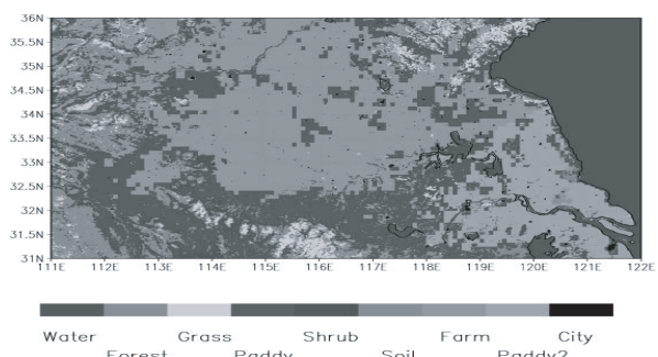
図 3：HUBEX の土地利用図 (変換後 2 期作地帯を追加)
