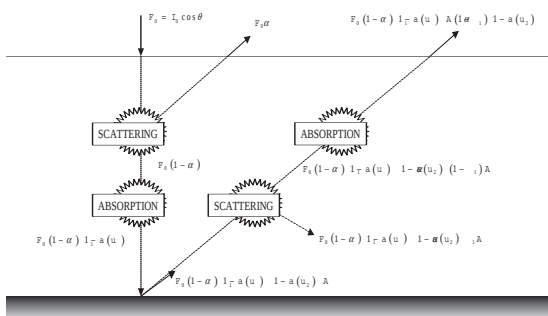
図 1：晴天モデルの概念図
