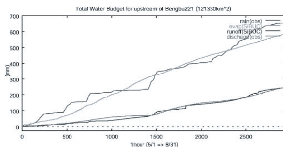
図6：蚌埠上流域でのSiBUCを用いた水収支推定(灌漑用水を考慮)
