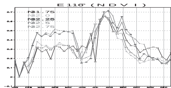
図 2：NDVI の時系列 (E116, 5 分メッシュ)
