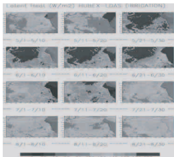
図5：HUBEX領域の潜熱フラックス分布(10日平均)
