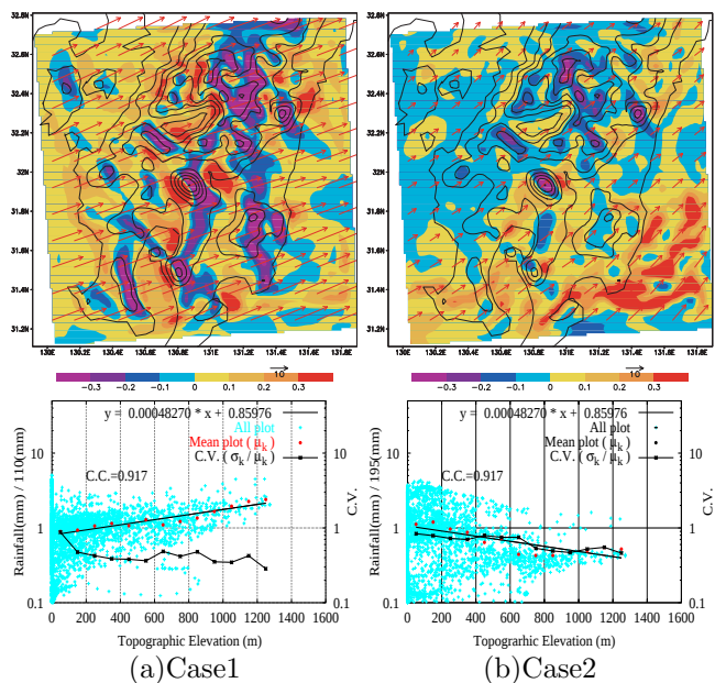
図3：2日間の平均上昇流および平均水平風速の分布（上図，単位は m/s）および地形標高と2日積算降雨量の関係（下図）（Case1：九州 98.6.13～14，Case2：九州 98.10.6～7）
