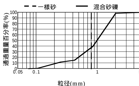
図-2 河床材料の粒度分布
