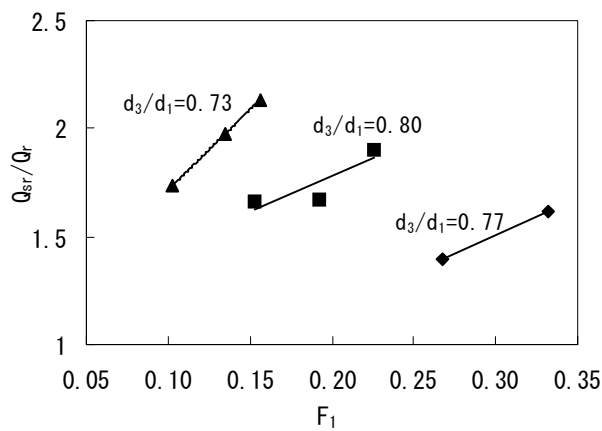
図-4(b) Q_{sr}/Q_r とフルード数の関係 (60°)
