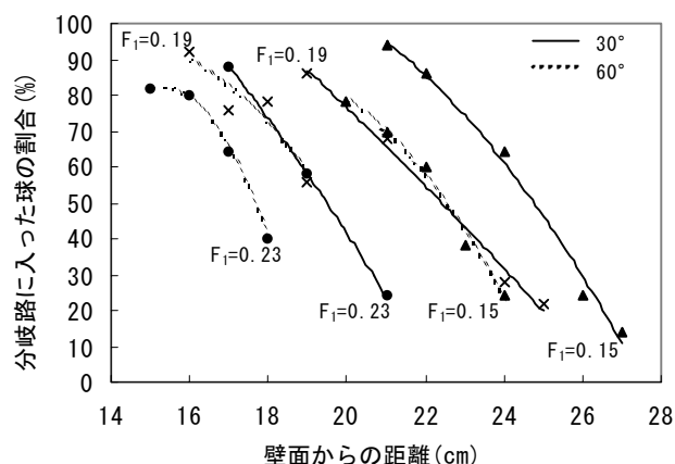
図-2 距離と入った球の割合の関係
