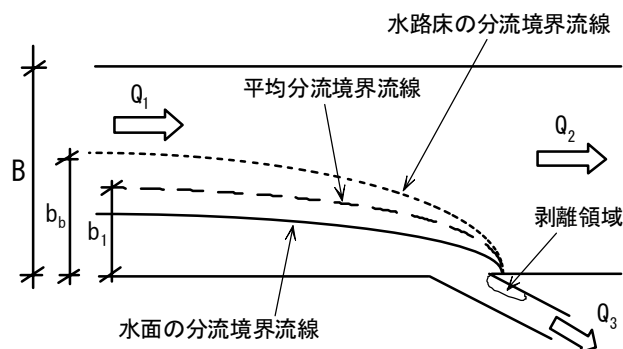
図-1 分岐部周辺の流れ
