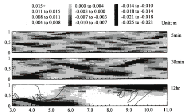
図2 流路形態の時間変化 (case2)
