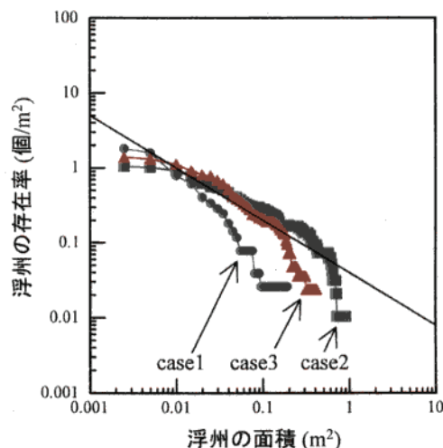
図5 浮州の面積とその面積以上の大きさを有する浮州の存在率との関係
