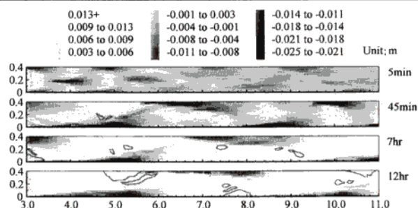
図1 流路形態の時間変化 (case1)
