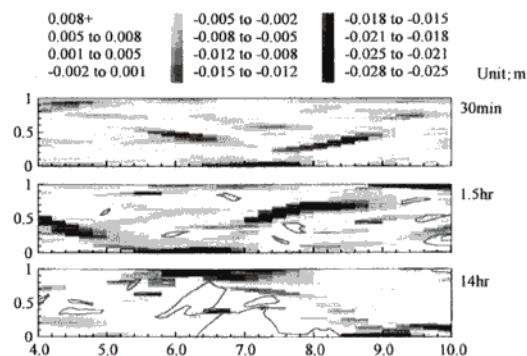
図3 流路形態の時間変化 (case3)
