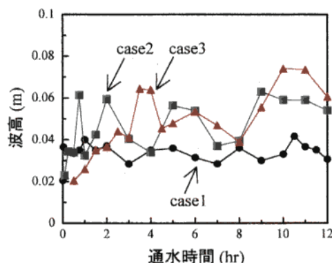
図4 波高の時間変化
