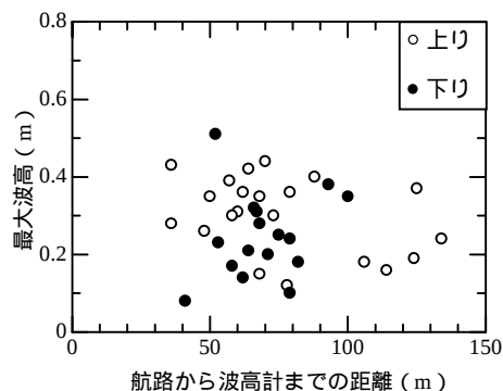
図-4 タンカーが造る航走波の特性
