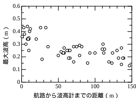
図-3 プレジャーボート型船が造る航走波の特性
