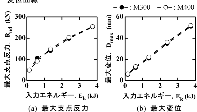
図-4 各種応答値と入力エネルギーの関係
