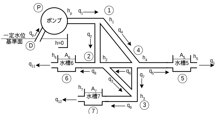
図1 ポンプと水槽を含む管網系モデル
