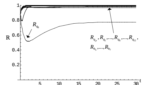
図5 センサの信用度の変化
