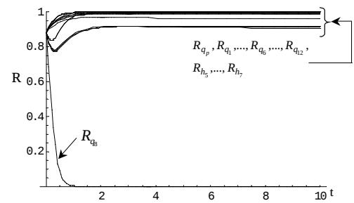
図3 センサの信用度の変化
