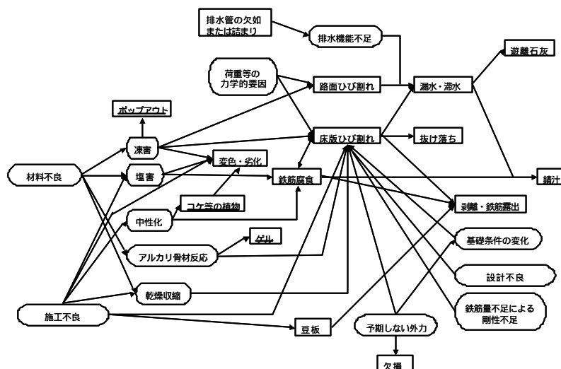
図1 変更後の床版に対する因果ネットワーク
