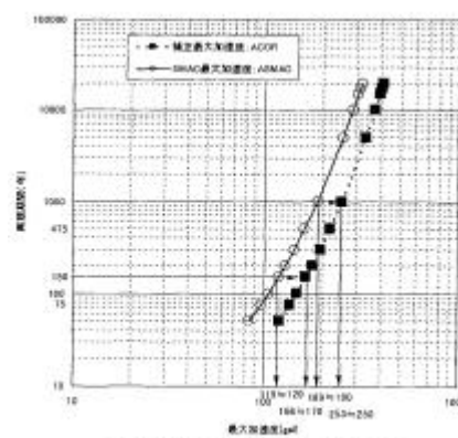
図-2 最大加速度と再現期間
