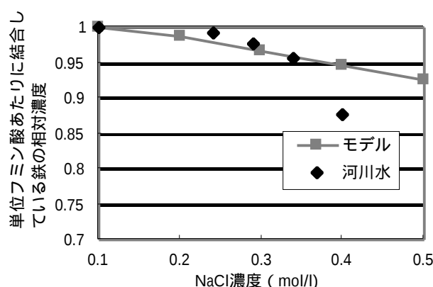
図 4. 0.1 \text{ mol/l} NaCl での鉄濃度を 1 とした時の競合を考慮した平衡モデルによる結果と河川水測定結果
