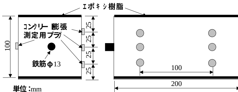
図 1 供試体図
