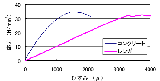
図2 圧縮試験における応力－ひずみ曲線
