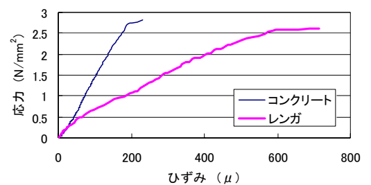
図3 割裂試験における応力－ひずみ曲線
