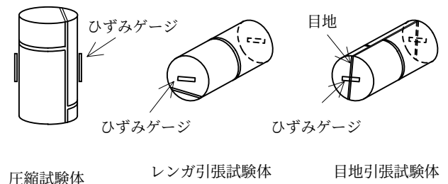
図 1 試験体概要図
