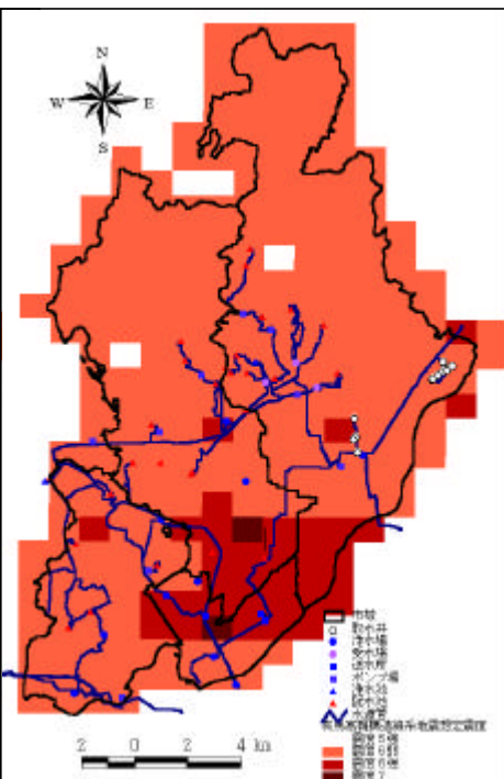
図5 水道ネットワークと有馬・高槻 構造線系地震想定震度 4)
