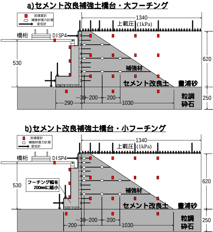
図1 橋台模型、計測機器配置の概略図
