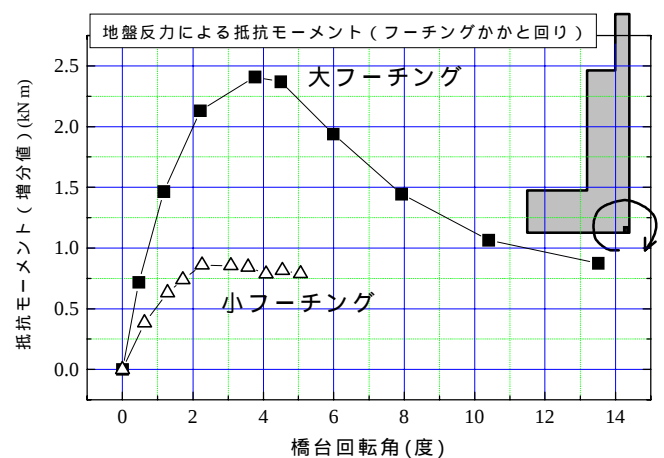
図 4 地盤反力による抵抗モーメントと橋台回転角の関係
