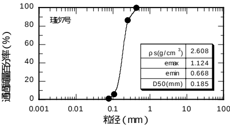
図-2 珪砂 7 号の粒度分布
