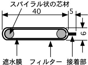
図-3 非排水性 PBD の形状
