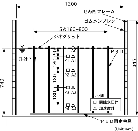
図-1 振動台実験装置
