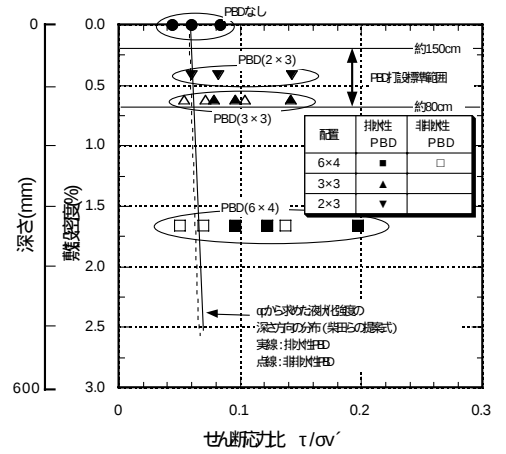
図-5 地盤の液状化強度
