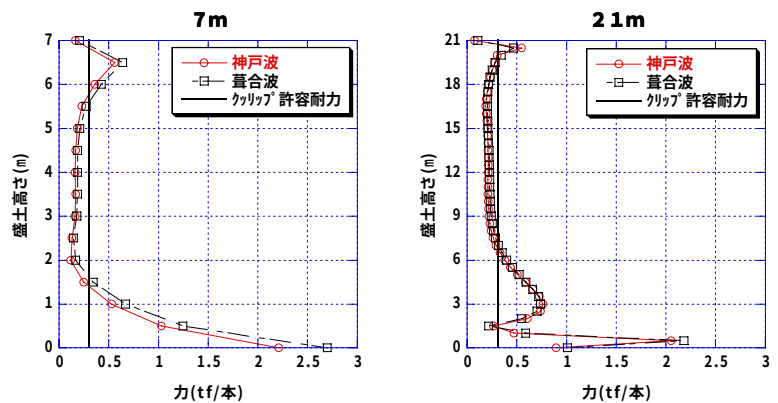
図-5 保護壁を支持している金具に働く力
