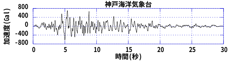
図-3 入力地震動
