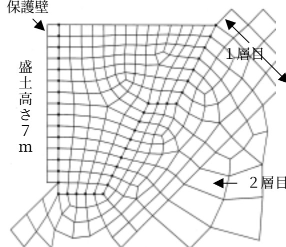
図-2 高さ 7m の軽量盛土部の FEM モデル
