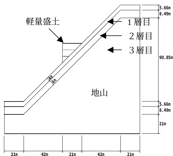
図-1 解析モデルの概要
