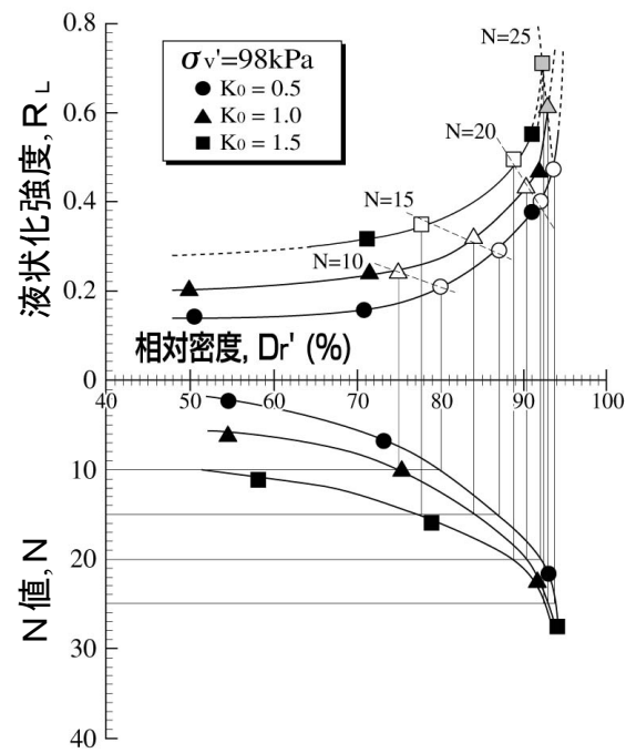
図-4 N値～相対密度～液状化強度の関係
