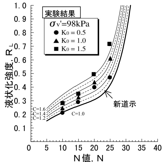
図-5 N値と液状化強度の関係
