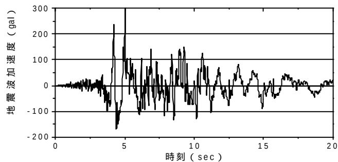
図-2 入力地震波 (NS 成分)
