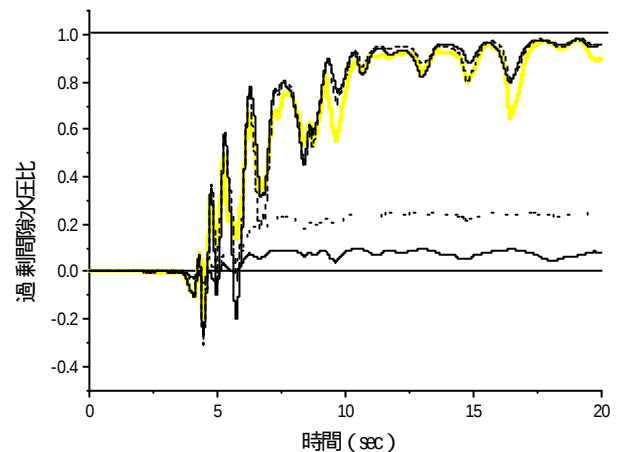
図-6 過剰間隙水圧比の時刻歴
