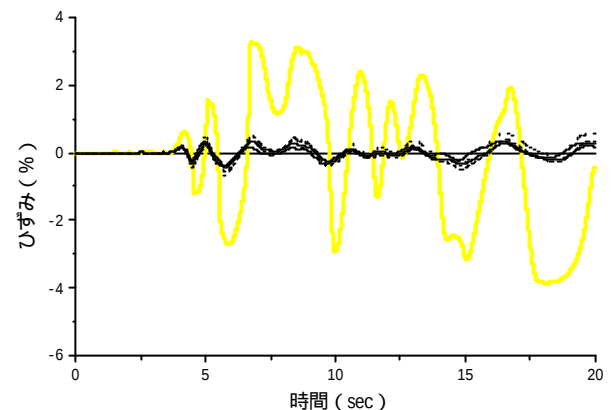
図-5 せん断ひずみの時刻歴
