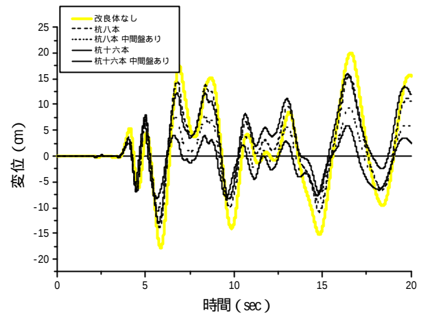
図-4 変位の時刻歴
