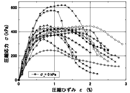
図-5 遅延载荷した場合の応力・ひずみ関係
