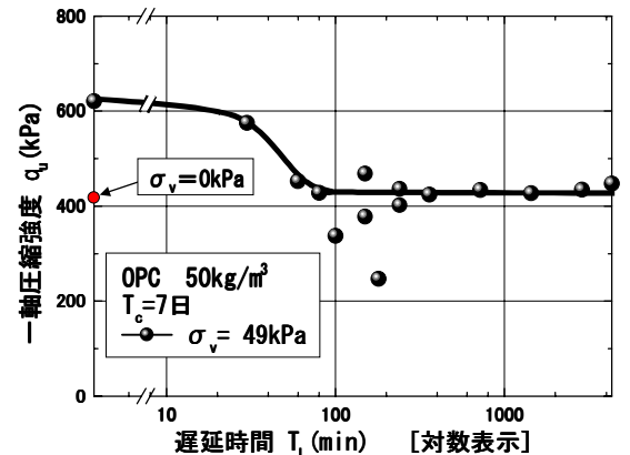
図-6 遅延载荷時間と一軸圧縮強度の関係
