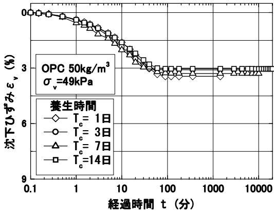
図-1 養生時間が異なる場合の沈下ひずみと経過時間の関係
