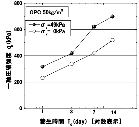
図-3 養生時間と一軸圧縮強度の関係
