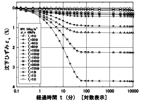
図-4 遅延载荷した場合の沈下ひずみと経過時間の関係
