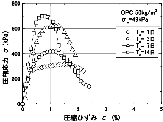
図-2 養生時間が異なる場合の応力と圧縮ひずみの関係
