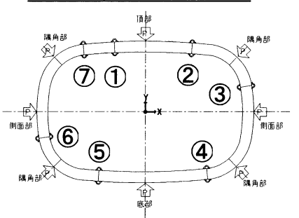
図 4 継手およびクリップゲージ設置位置
