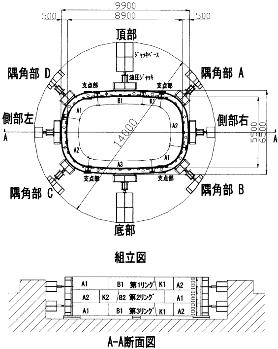
図1 供試体形状と載荷状況図
