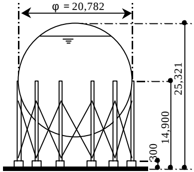
図-1. 検討対象構造物
