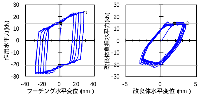
図-8. 鉛直荷重 80kN 時の結果(大変形領域)
