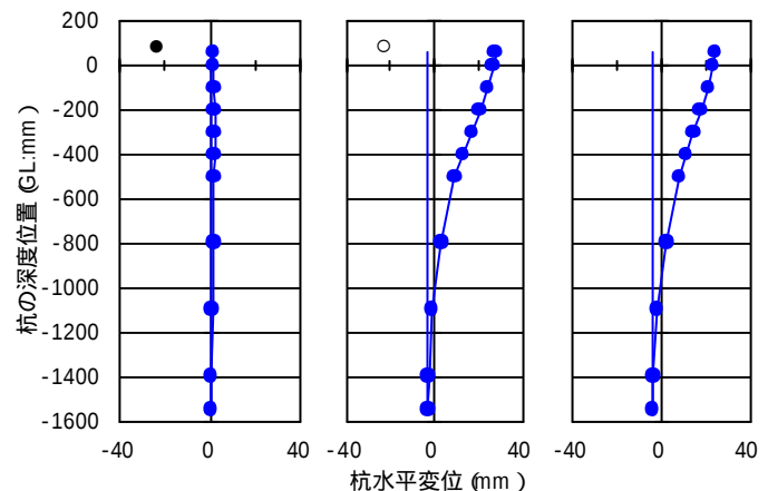
図-9. 杭の深度方向の変位分布
