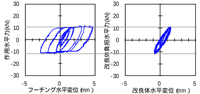
図-6. 鉛直荷重 40kN 時の結果(小変形領域)
