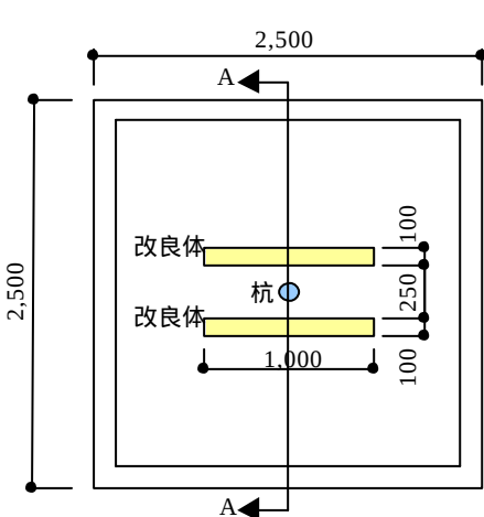
図-3. 試験体平面図
