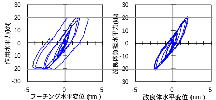
図-7. 鉛直荷重 80kN 時の結果(小変形領域)
