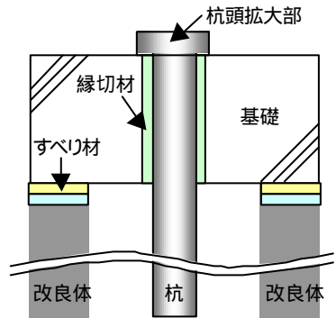
図-2. 杭頭模式図
