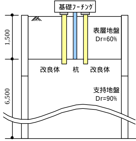
図-4. A-A断面図
