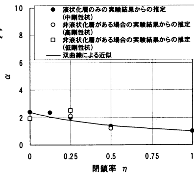
図-4 \alpha と閉鎖率 \eta の関係(液化化層)
