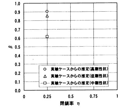
図-5 \beta と閉鎖率 \eta の関係(液化化層)
