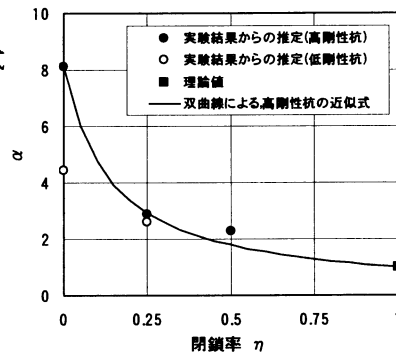
図-2 \alpha と閉鎖率 \eta の関係(非液化化層)
