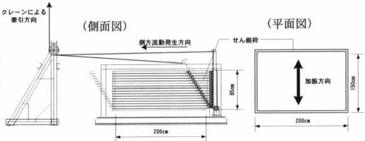
図-1 せん断土槽概要図
