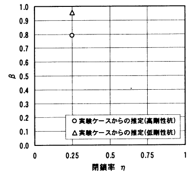
図-3 \beta と閉鎖率 \eta の関係(非液化化層)
