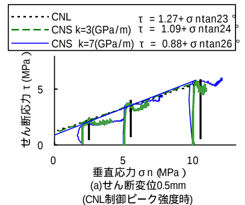
図 - 4 試験結果( \sigma_{n0}=5\text{MPa} )
