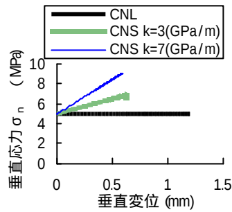
図 - 3 垂直応力の制御結果
