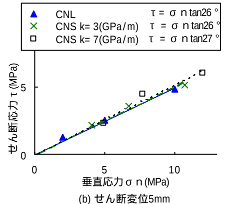
図 - 5 せん断試験の応力経路
