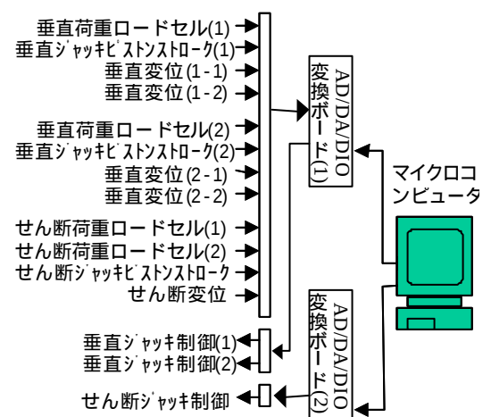
図-2 デジタル制御システム構成
