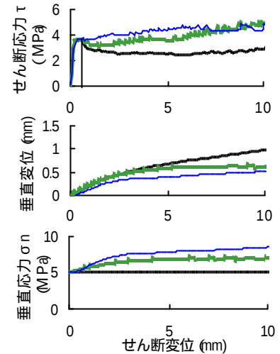
図 - 4 試験結果( \sigma_{n0}=5\text{MPa} )
