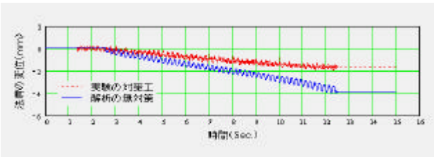
図－4 法肩の変位時刻歴（対策）
