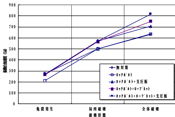
図-2: 破壊形態と振動台加速度
