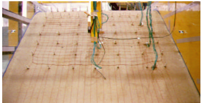
写真-1:ロックボルトとロープネットによる対策工
