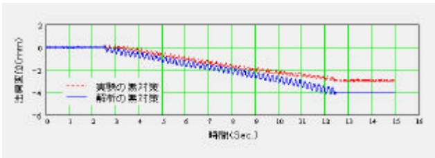
図－3 法肩の変位時刻歴（無対策）
