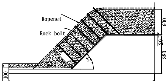
図-1 :斜面の対策工
