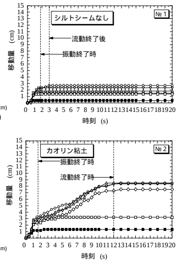
図-4 移動量の時刻歴
