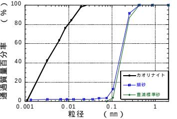
図-2 粒径加積曲線
