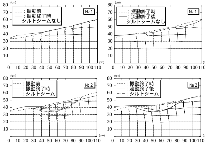
図-3 流動の様子
