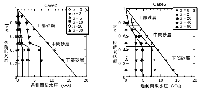
図-4 過剰間隙水圧の時間的変化
