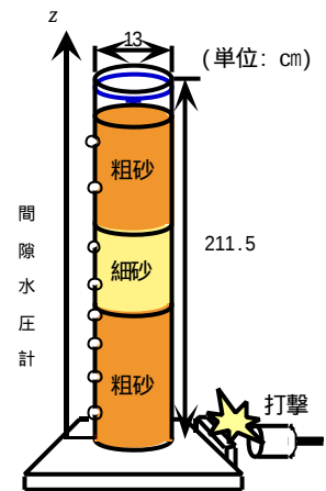
図-1 実験装置
