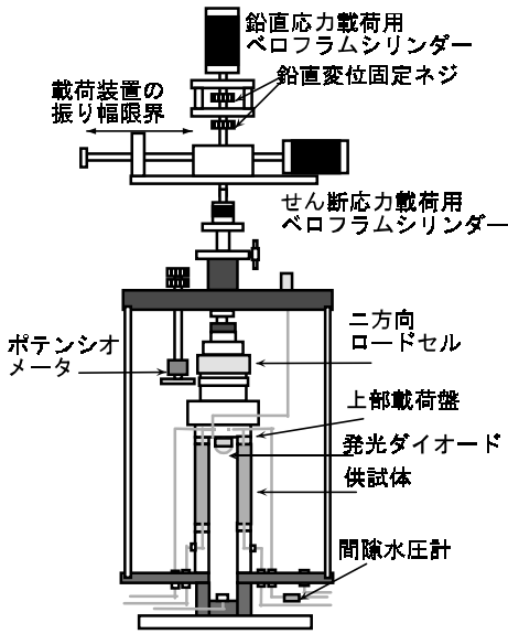
図1 試験機概要
