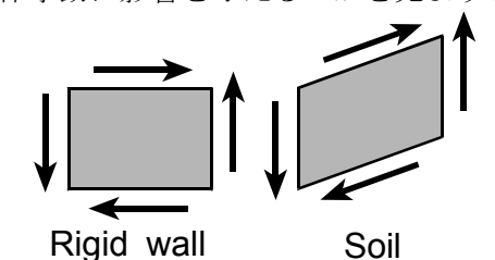
図-1 剛壁に隣接する土要素の挙動
