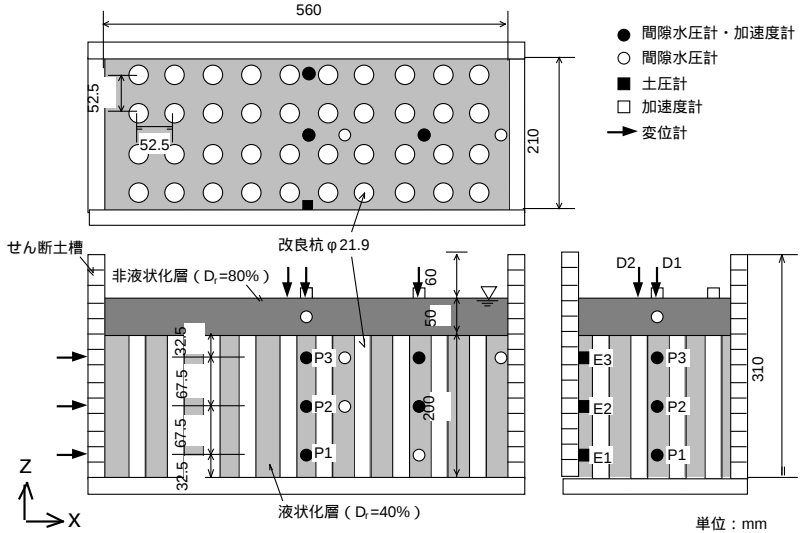
図-1 実験モデルおよびセンサー設置位置
