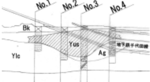
図 - 4 液状化層の分布状況
