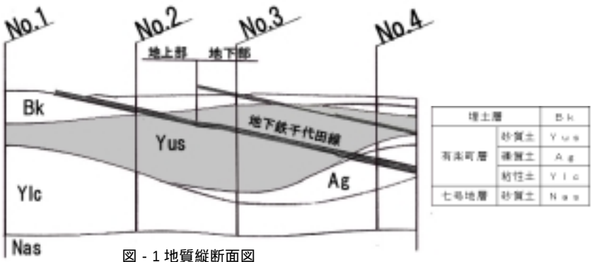
図 - 1 地質縦断面図
