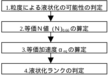
図 - 3 港湾施設基準による液状化判定フロー
