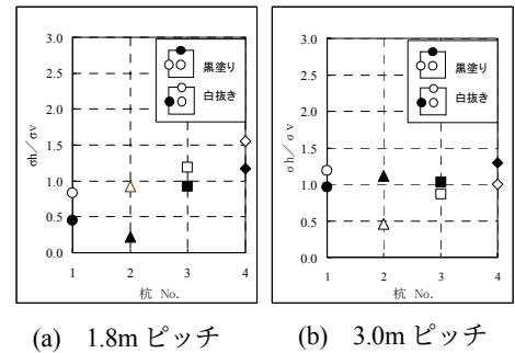
図-5 拡張終了時の k 値 ( \sigma_h'/\sigma_v ) (実験 1,4)
