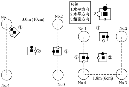
図-2 計測位置
