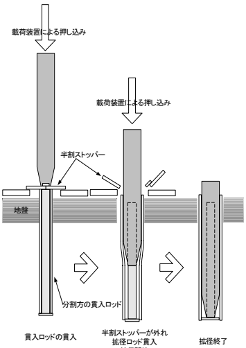
図-1 ロッド貫入と拡張順序
