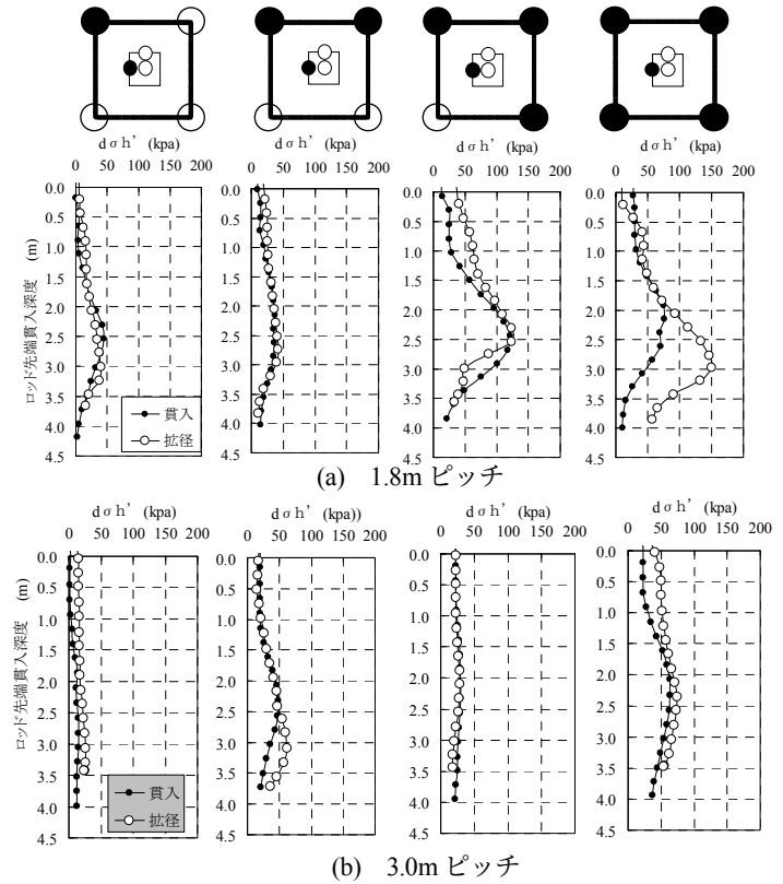
図-4 貫入・拡張時地盤内水平有効土圧増分（実験 1、4）
