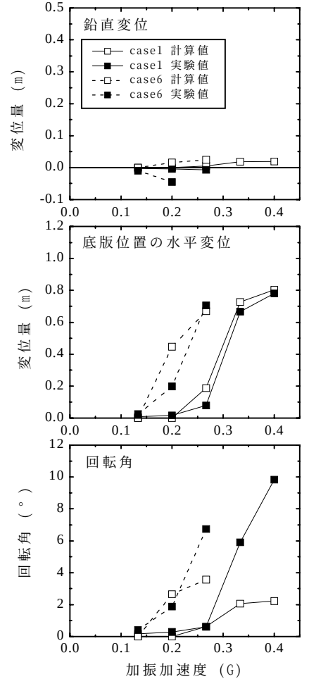
図-4 加振加速度と変位量 ( \mu=0.57 、 \psi=0.45 )
